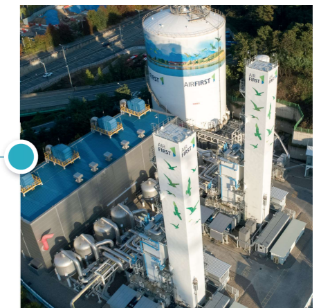
용인공장 2 N2 Generator 반도체 산업단지
